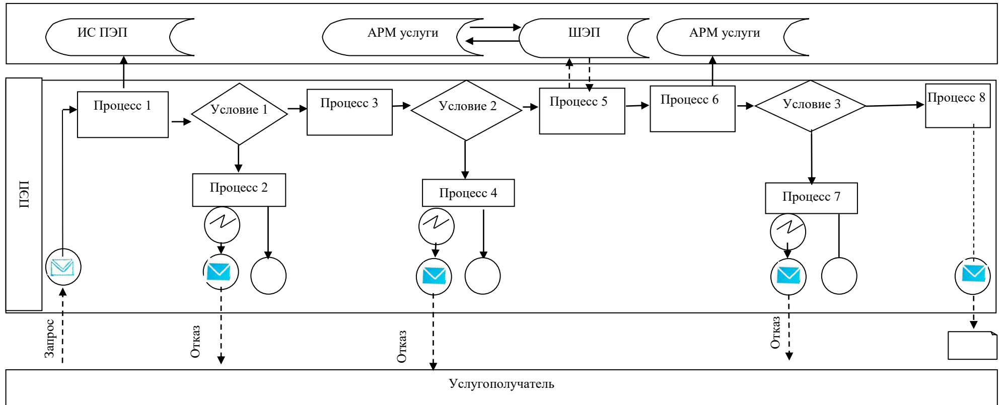
Диаграмма функционального взаимодействия информационных систем, задействованных в оказании государственной услуги через портал
